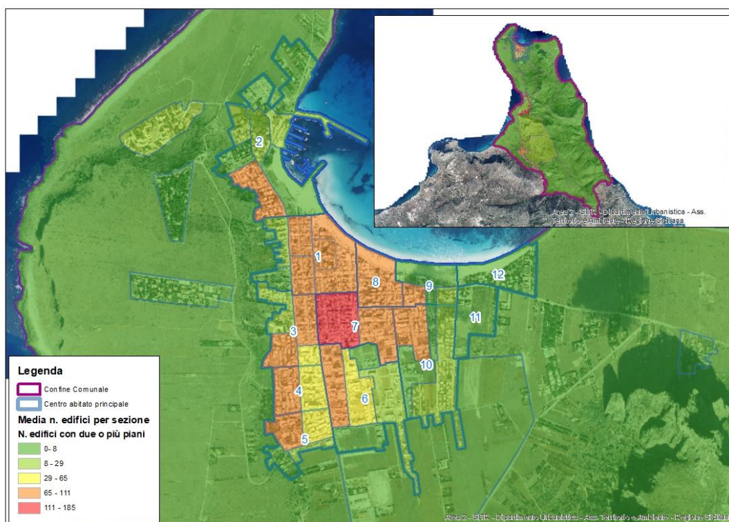
Figura 16 - distribuzione media edifici con due o più piani
