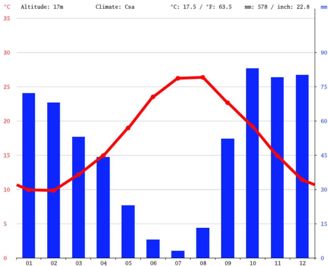
Figura 21 - Grafico delle temperature e delle precipitazioni medie mensili
