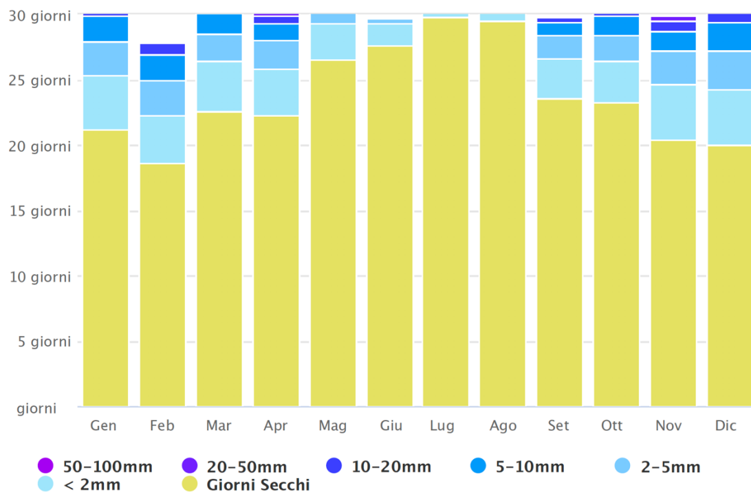
Figura 23 – Quantità di precipitazione
