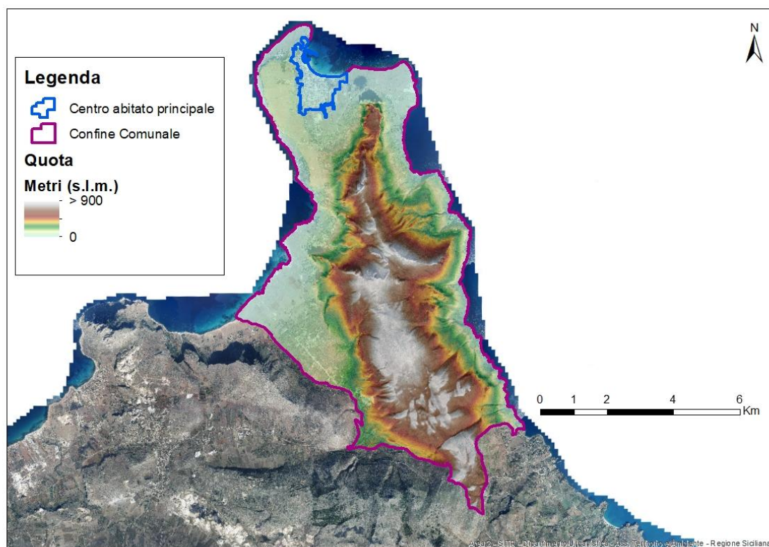
Figura 17 - Carta delle altimetrie
