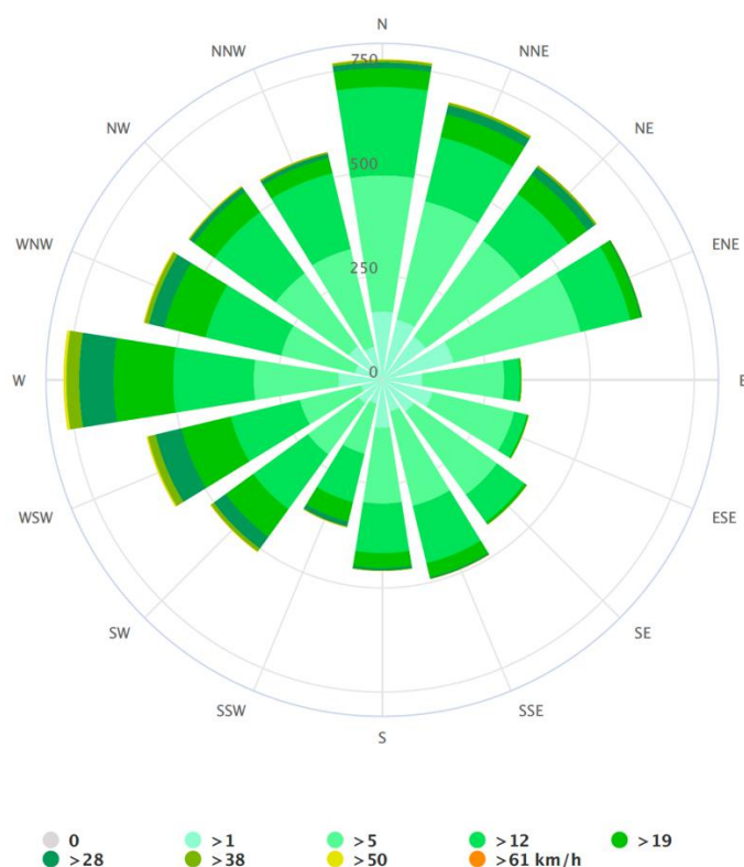
Figura 25 - Rosa dei venti
