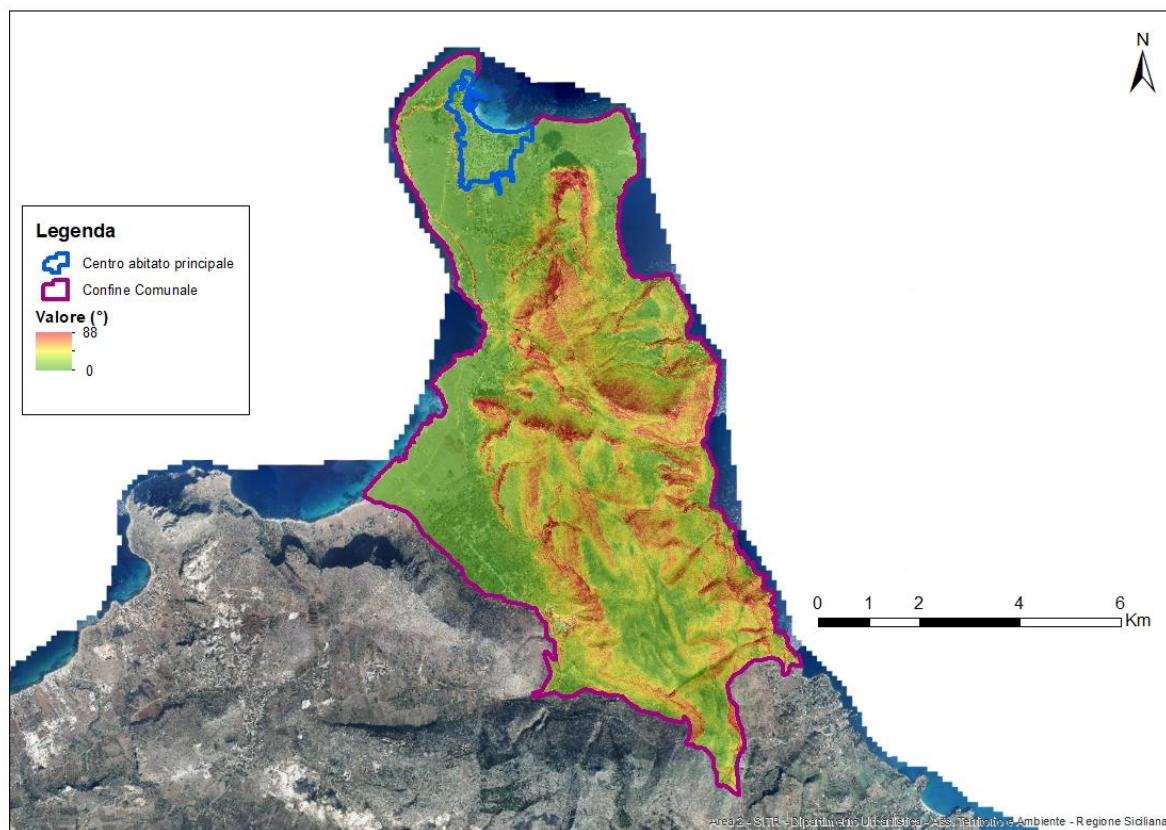
Figura 18 – Carta delle pendenze
