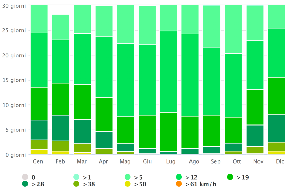
Figura 24 - Velocità dei venti
