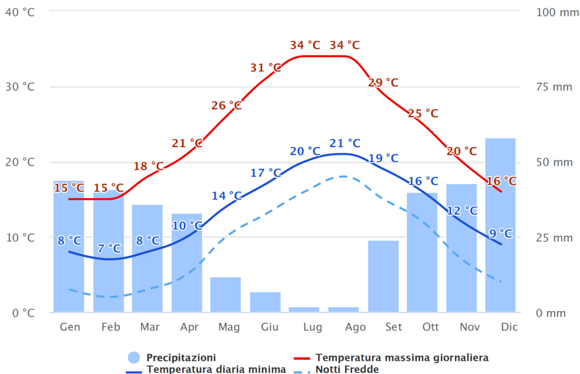
Figura 20 - Temperature e precipitazioni medie giornaliere
